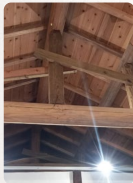
▲ 左圖「在來軸組工法」的屋體結構，右圖「簾子下見」式的雨淋板 / 陳文彥
