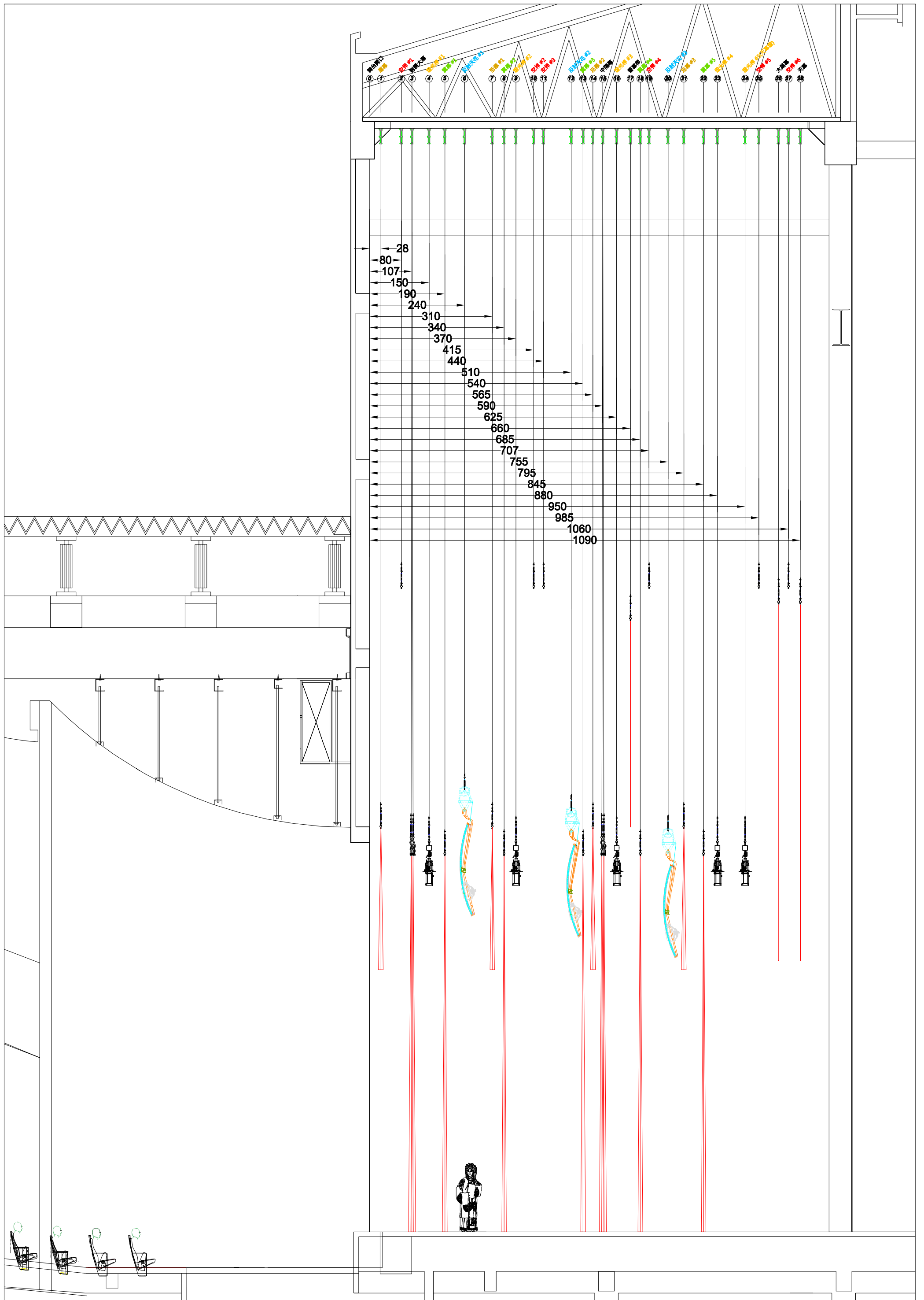
新營文化中心演藝廳 側視圖 (單位:cm)
