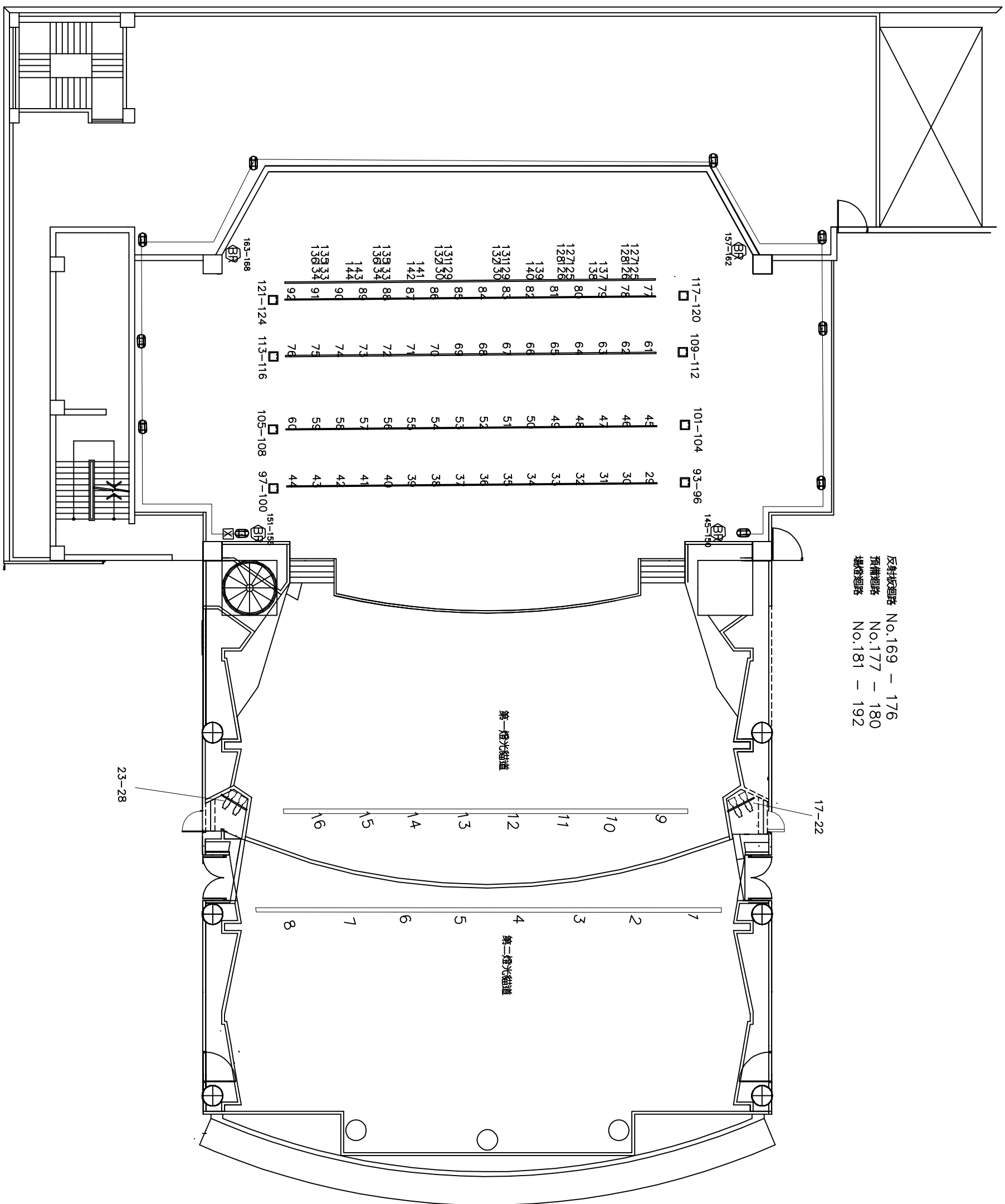
新營演藝廳燈光迴路配置圖
